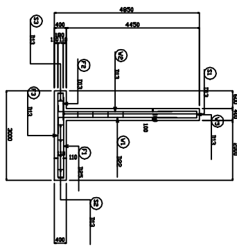
断面図 S=1:60
