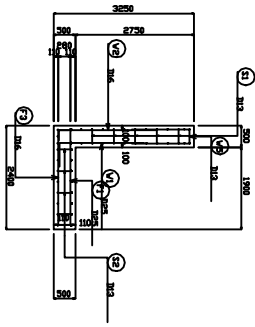
断面図 S=1:60
